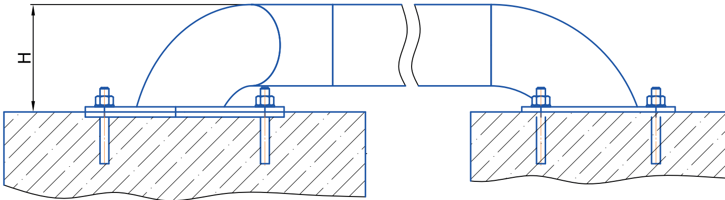
А-А (вариант 2)
